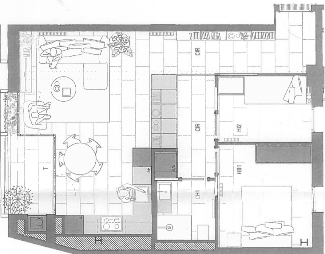
PLANTA BAIXA
