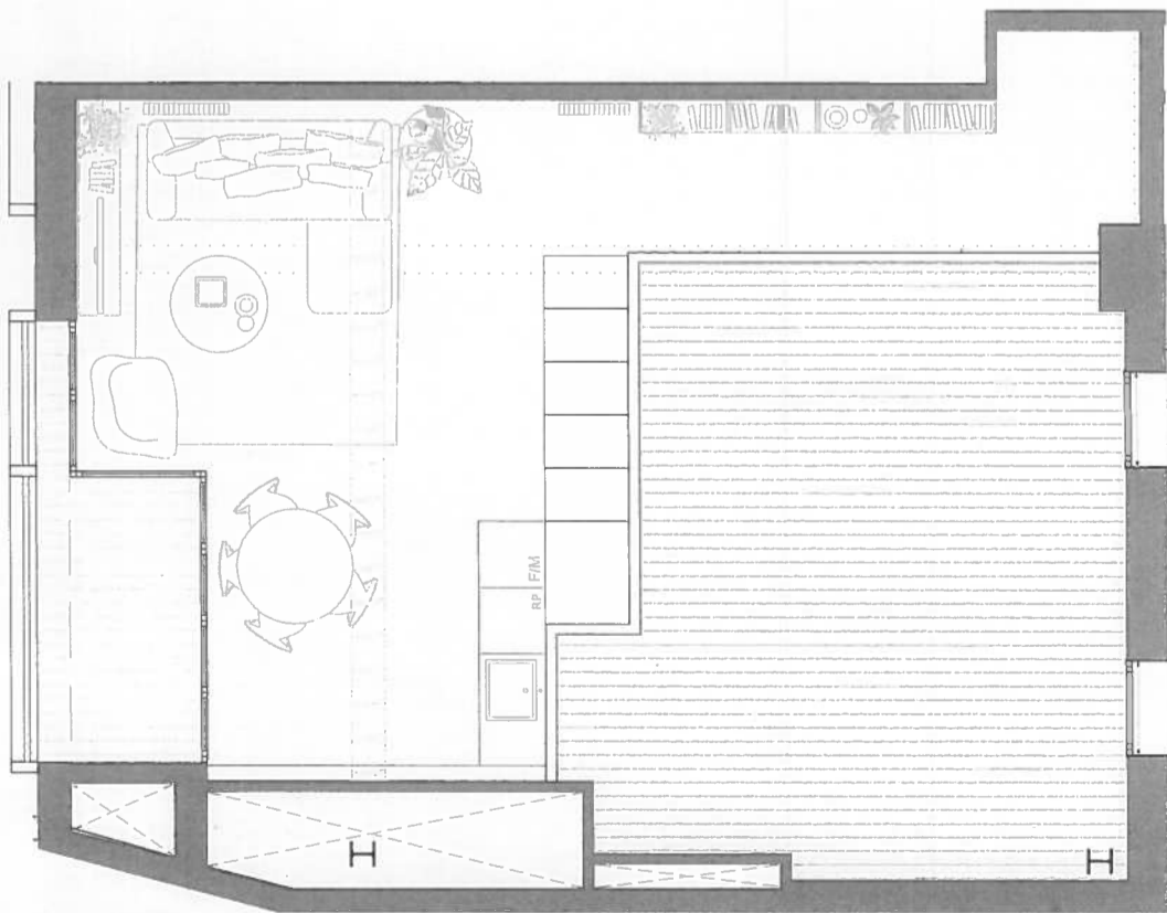
PLANTA ALTELL
